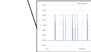
SCLK
