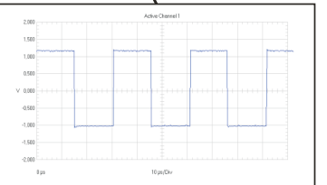
32 kHz SLEEPCLK
