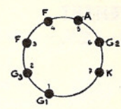
EF 93 6BA 6
