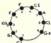
EL84-6BQ5
