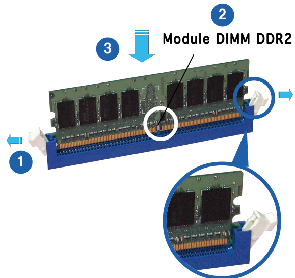
Clip de rétention déverrouillé
